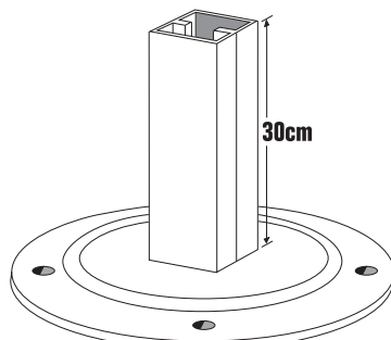
ANCLAJE POSTE OCTOGONAL 4 GUÍAS
